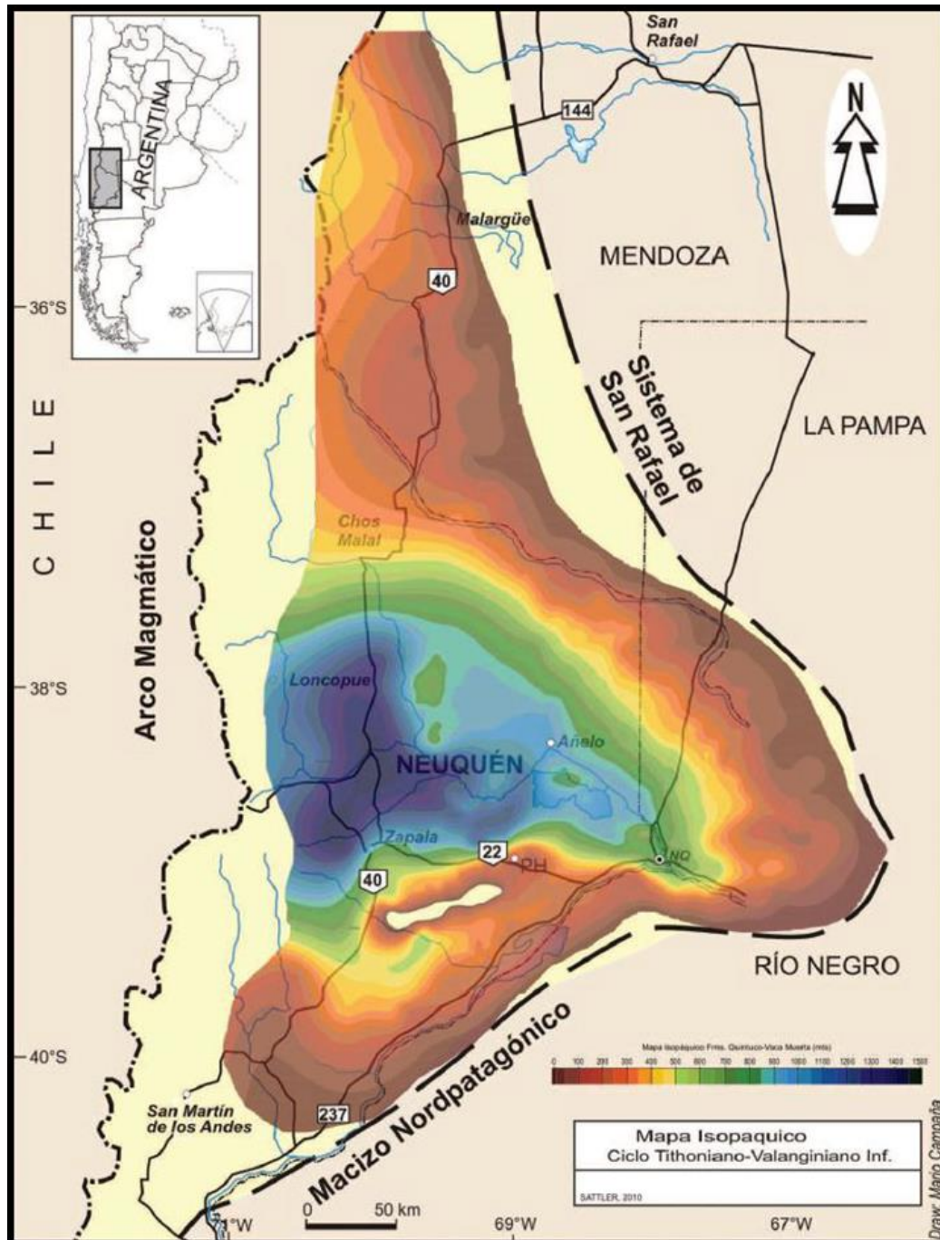
Mapa isopáquico del ciclo Tithoniano a Valanginiano Temprano en la Cuenca Neuquina. De la Publicación "LA FORMACIÓN VACA MUERTA Y EQUIVALENTES (JURÁSICO TARDÍO-CRETÁCICO TEMPRANO) EN LA CUENCA NEUQUINA" Autores: Héctor A. Leanza, Federico. Sattler, Ricardo S. Martínez y Osvaldo Carbone Expuesto en el RELATORIO DEL XVIII CONGRESO GEOLÓGICO ARGENTINO • NEUQUÉN, 2011
